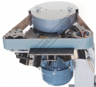
Optional Platen Table (L097)
