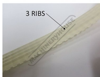
BP252 POLY RIB BELT.2
